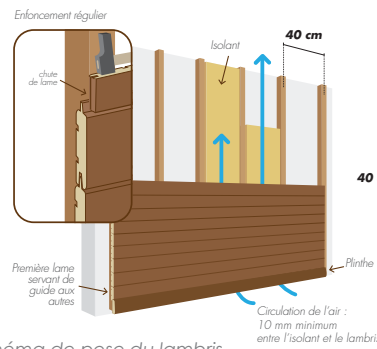
Schéma de pose du lambris
